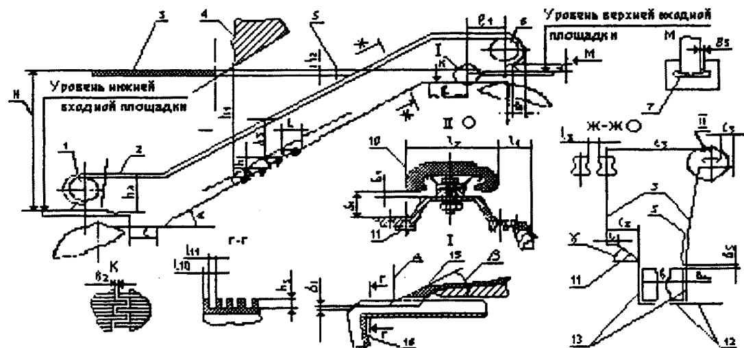
Рисунок 1. Схема устройства эскалатора
